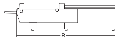
Protezione cilindro e valvole sfiato aria tampone Cylinder protection and pad exhaust valves
