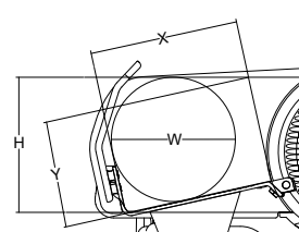
Tubo per taglio verdure mm Ø200 h.345 Vegetables cùte
